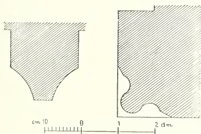
Obr. 169. Ranná. Profil portálu a žebor.
