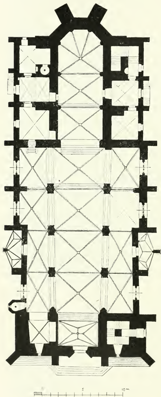
Obr. 31. Chrudim. Půdorys kostela hlavního.
