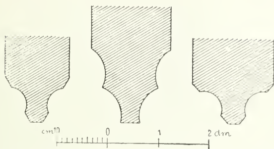
Obr. 66. Chrudim. Kostel sv. Kateřiny; Profily žebel v choru, lodí a sakristii.
