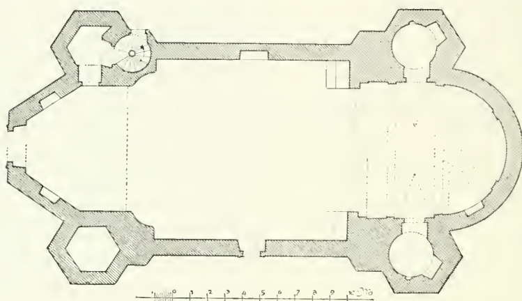
Obr. 165. Podskalí. Kaple sv. Jana Křtitele.
