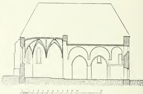
Obr. 135. Kostelec u Městce. Kostel sv. Petra a Pavla; řez podélný
