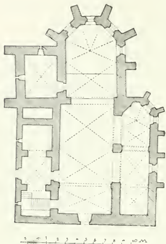
Obr. 134. Kostelec u Městce. Kostel sv. Petra a Pavla.
