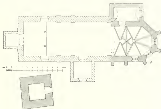
Obr. 141. Líciborice. Půdorys kostela sv. Michala.
