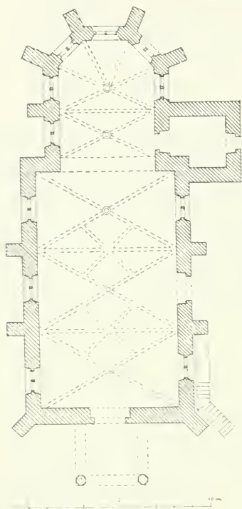
Obr. 74. Chrudim. Kostel sv. Michala.
