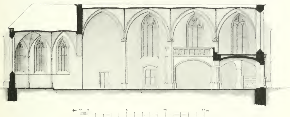
Obr. 64. Chrudim. Kostel sv. Kateřiny; řez podélný (před poslední opravou).
