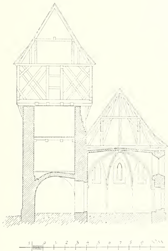
Obr. 160. Morašice. Řez kostela, vazba věže před opravou.
