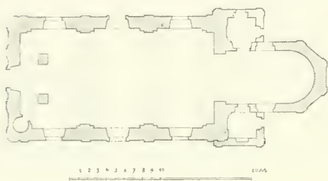
Obr. 2. Bojanov. Kostel sv. Víta.
