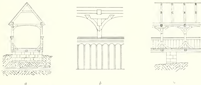
Obr. 125. Kočí. Most kostelní; a , c řez příčný a podélný, b pažení a vazba trámů.
