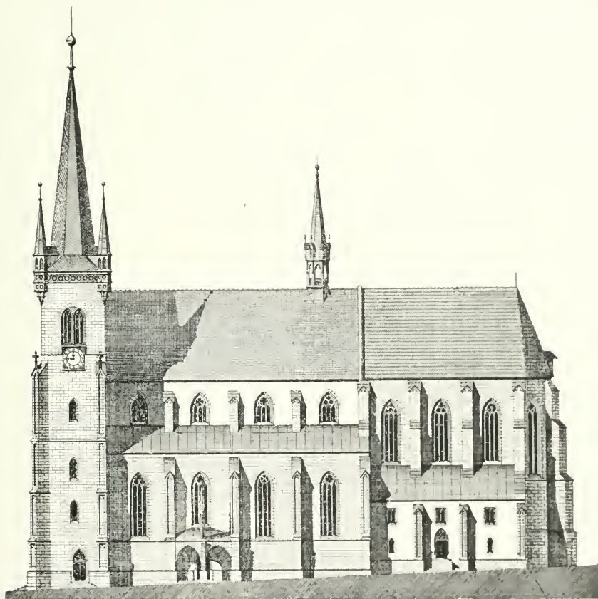
Obr. 32. Chrudim. Kostel hlavní, strana jižní.
